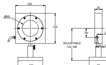
L50(300)A-LP2-65
