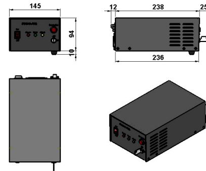
236(L)×145(W)×104(H) mm 3 , 2.3 kg
