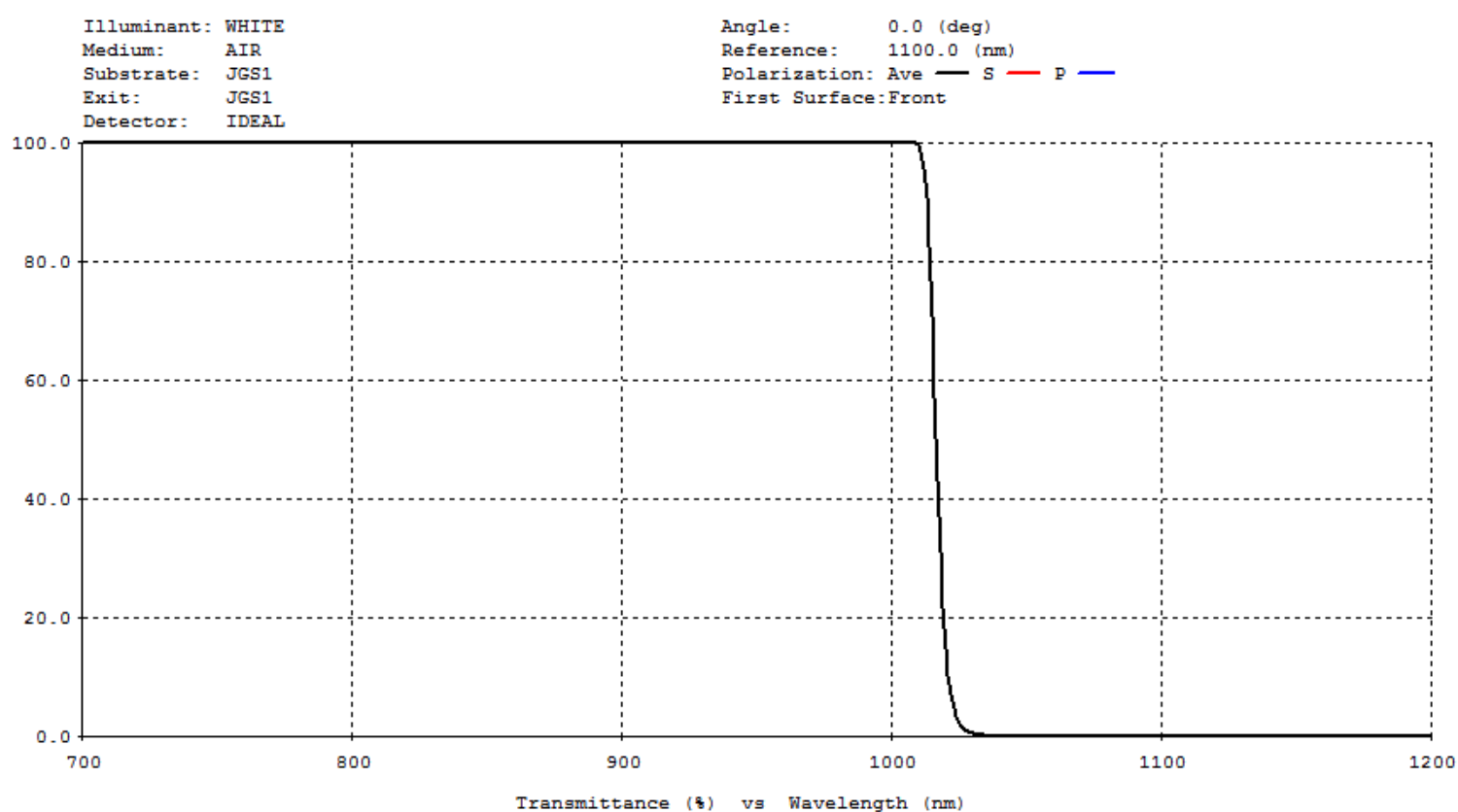
HR@1050-1150nm & HT@780-980nm AOI=0°
