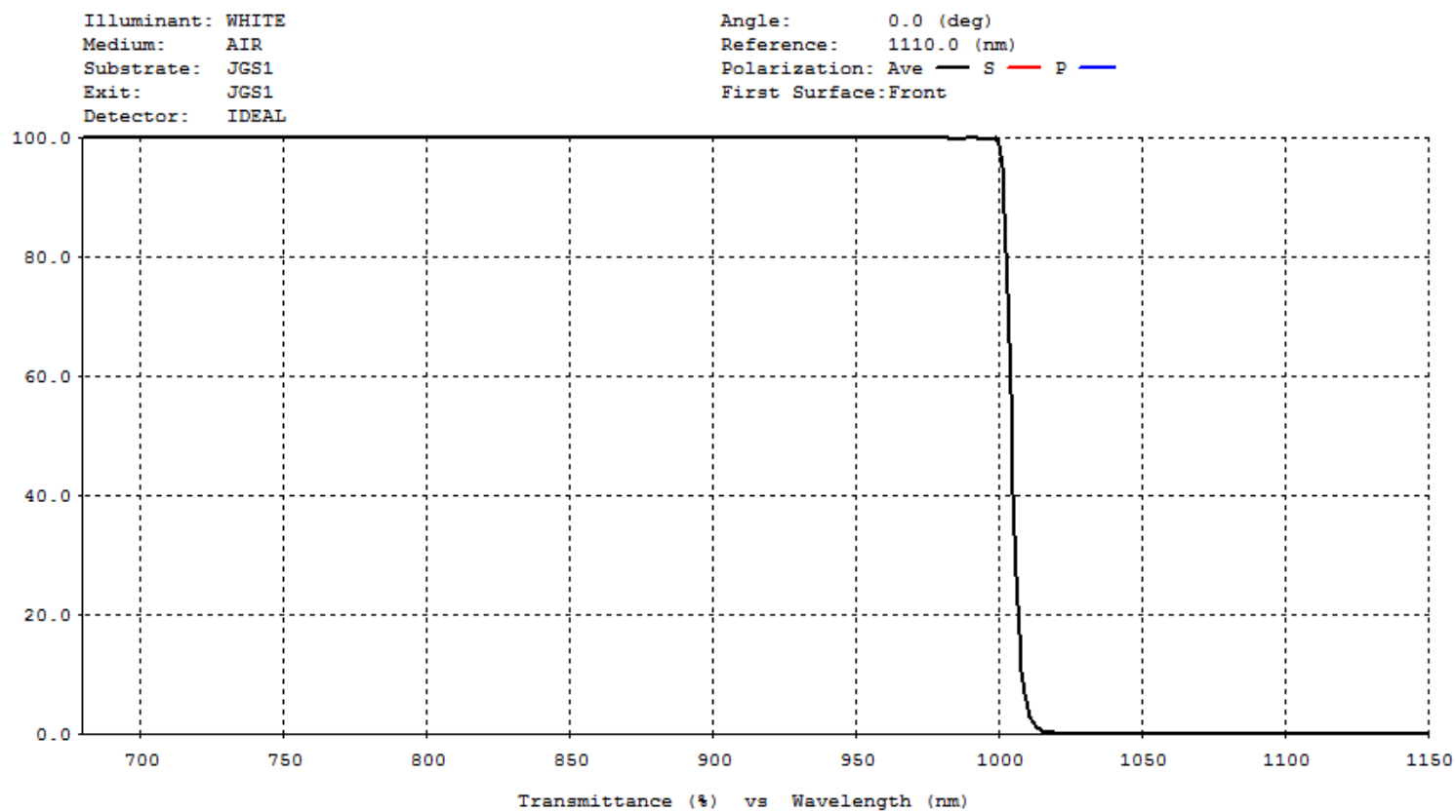
HR@1030-1100nm & HT@700-1000nm AOI=0°
