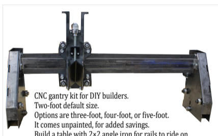
DIY CNC Gantry Kit
