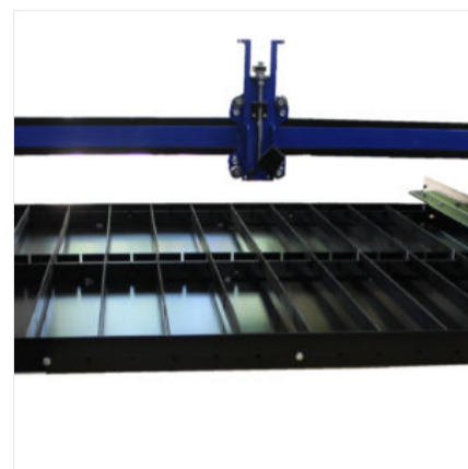
4x8 expandable CNC plasma table
